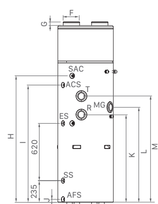
VISTA TRASERA HYDREA 280
