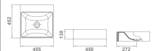
10221 ALBUS 45 x 45 cm €/u 12,5 32 139,0 Sin rebosadero. Sin orificio de grifería. Esmaltado por los cuatro lados.
