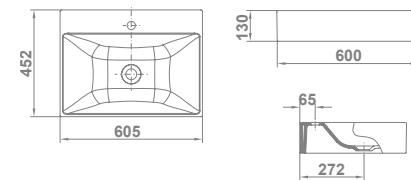
10215 ALBUS 60 x 45 cm €/u 15 32 164,5 Sin rebosadero. Con orificio de grifería. Esmaltado por los cuatro lados.
