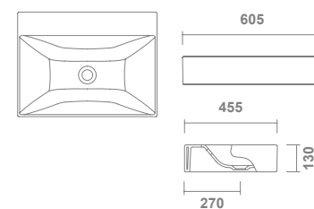
10217 ALBUS 60 x 45 cm €/u 16 32 164,5 Sin rebosadero. Sin orificio de grifería. Esmaltado por los cuatro lados.
