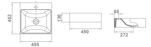
10219 ALBUS 45 x 45 cm €/u 12,5 32 139,0 Sin rebosadero. Con orificio de grifería. Esmaltado por los cuatro lados.
